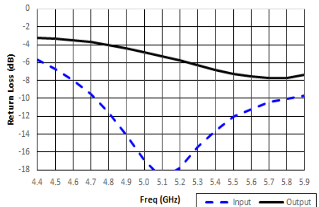
MGA-495940-02 Return Loss
