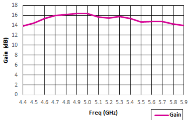
MGA-495940-02 Gain
